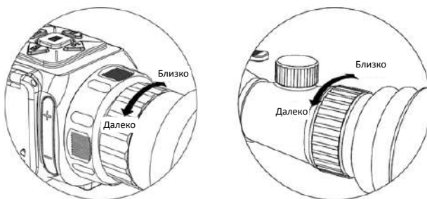
Рис. 3-1. Регулировка диоптра
