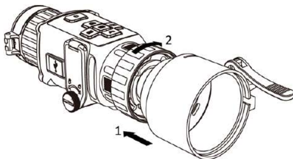
Рис. 2-4. Установка адаптера
