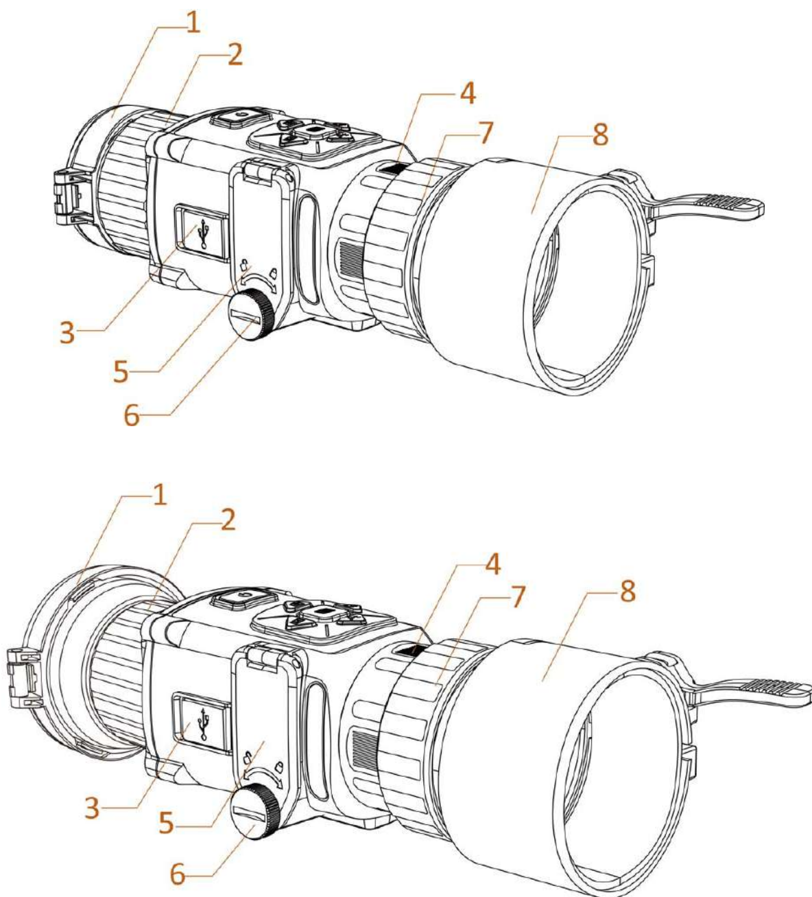
Рис. 1-2. Интерфейсы устройства
